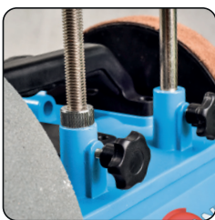
Support universel en F Ø12mm avec molette de réglage
