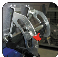
Guide en profilé aluminium inclinable à 45°
