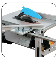
Loopwagen op gelijke hoogte met het blad
