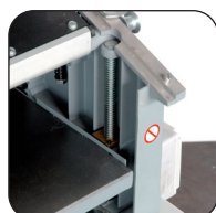
Schaafbank in gietstaal op 4 schroefvijzels
