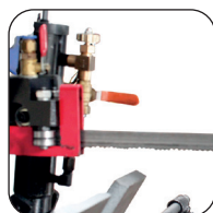
Aanpasbare en zeer nauwkeurige geleiding van het zaagblad met 8 punten rollen
