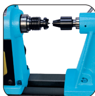
Meenemerstift met schroefdraad M33 x 3,5 mm
