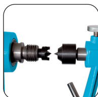
Meenemerstift CM2 schroefdraad M33 x 3,5 mm
