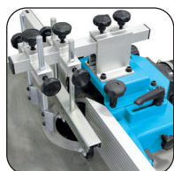
Guida toupie con pressore orizzontale e verticale
