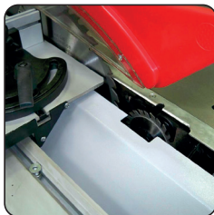
Lame Ø 315 inclinable à 45° et inciseur de 100mm
