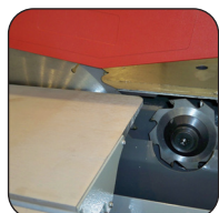
Zaagblad Ø 250 mm en voorritsblad Ø 80 mm
