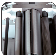
Schaafspindel van Ø 70 mm met 3 messen 310 x 25 x 3 mm
